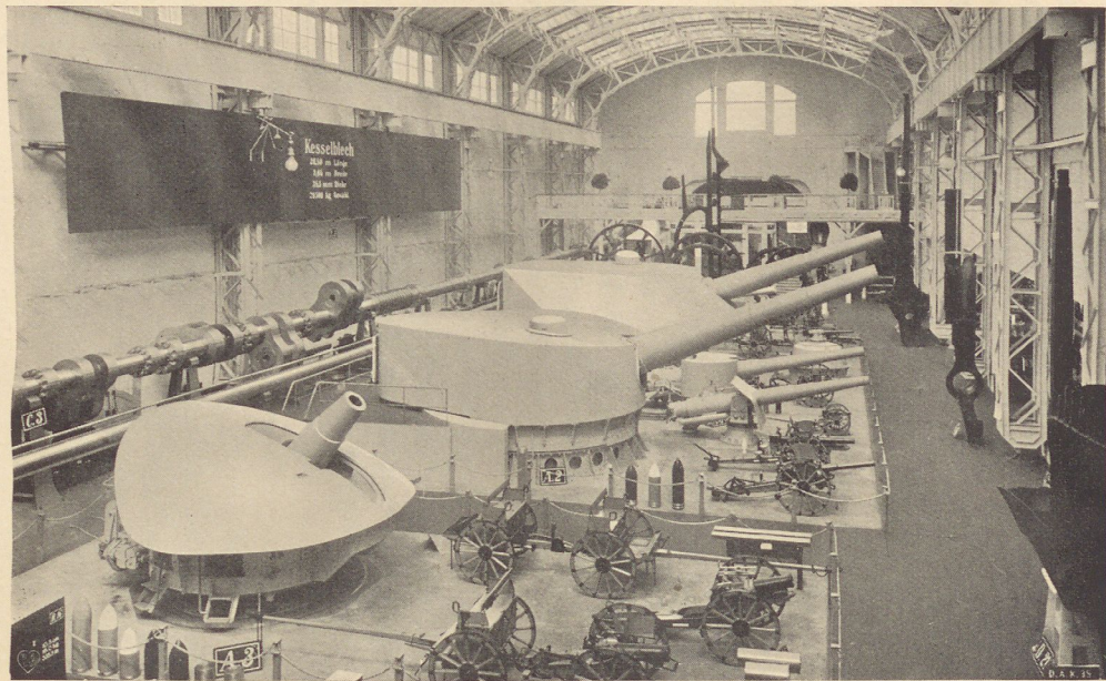
Kruppsches Artilleriematerial auf der Düsseldorfer Ausstellung 1902.
