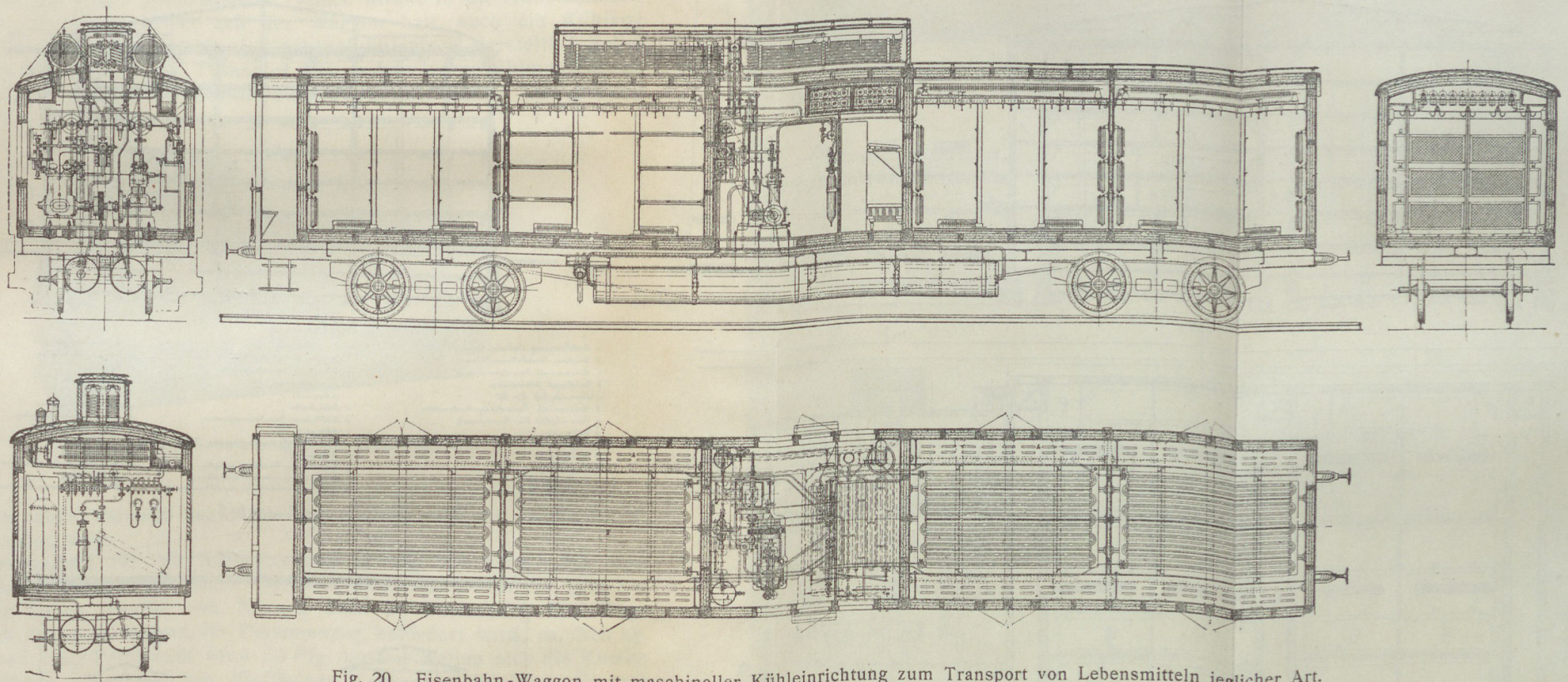
Fig. 20. Eisenbahn-Waggon mit maschineller Kühleinrichtung zum Transport von Lebensmitteln jeglicher Art. Ausgeführt für die russische Eisenbahn von der „Maschinenbau-Anstalt Humboldt in Köln-Kalk“.
