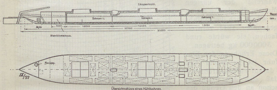
Fig. 30. Isolierter Kühlkahn (Grundriß u. Längsschnitt).
