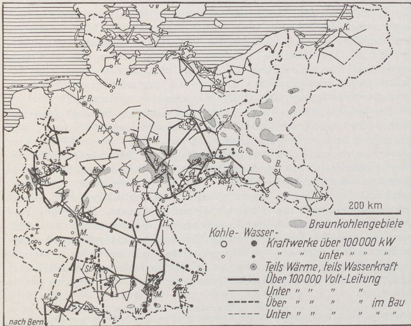
99. Die Großkraftleitungen im Deutschen Reich, März 1927.
