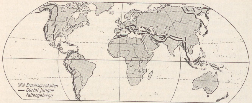
102. Verbreitung der Petroleumfelder und ihr Zusammenhang mit den geologischen Verhältnissen.
